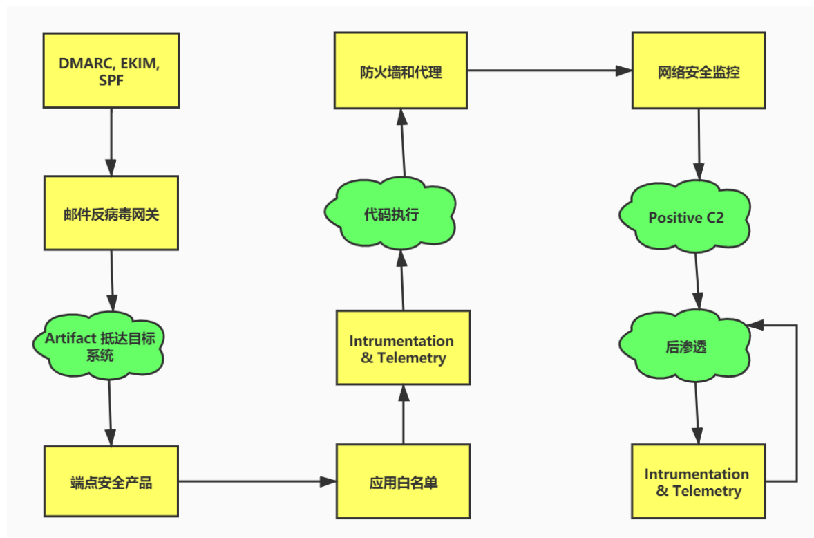
图1. 攻击问题集
